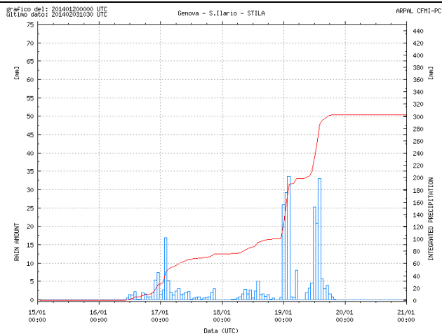
Figura 26 Ietogramma e cumulata di S. Ilario INTENSITA': (mm/1h, mm/3h) m. forte QUANTITA': (mm/6h, mm/12h, mm/24h) m. elevata
