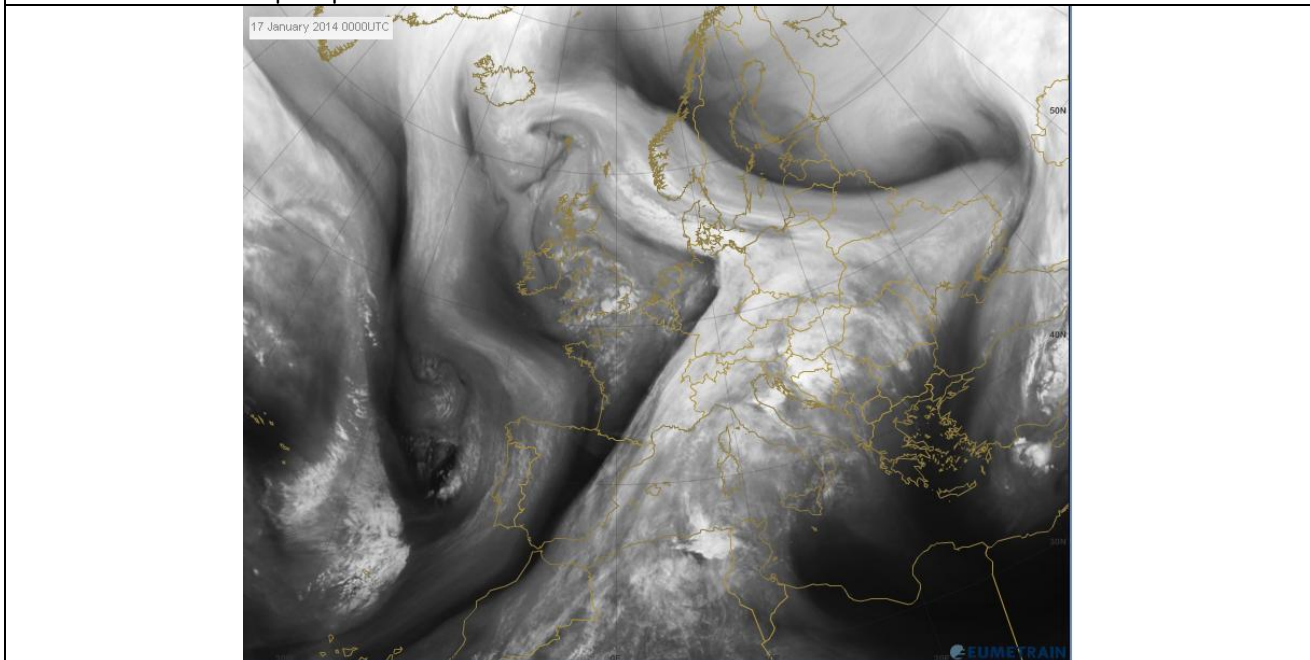
Figura 4 Immagine dal satellite MSG nel canale Water Vapor (WV6.2) riferita alle 00 UTC del 17 gennaio 2014 (elaborazione http://eumetrain.org/eport.html ): in evidenza l'imponente avvezione di aria umida dall'Atlantico e dall'Africa subtropicale verso l'Europa centrale.
